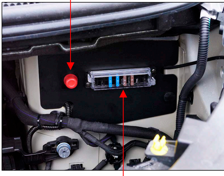
TAXI -Sicherungskasten
